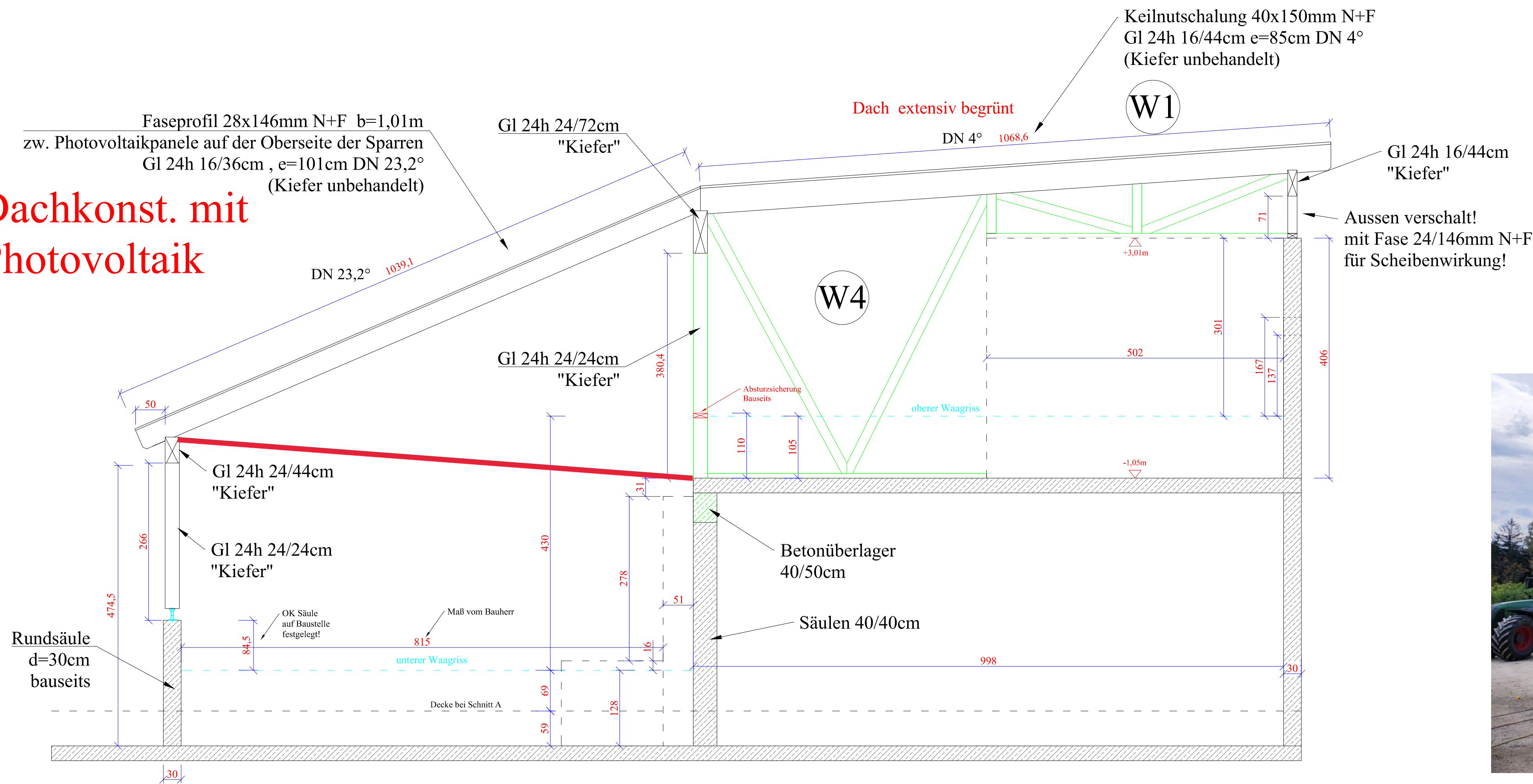
Schnitt B
