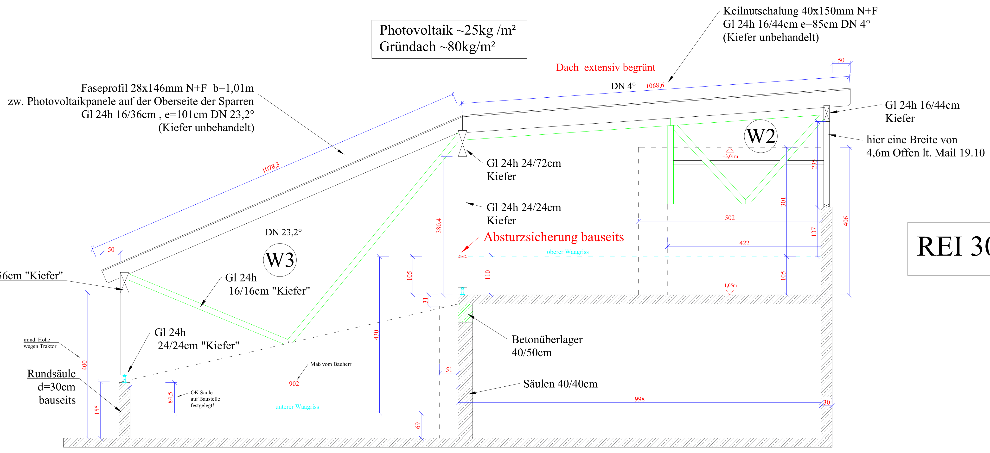
Schnitt A
