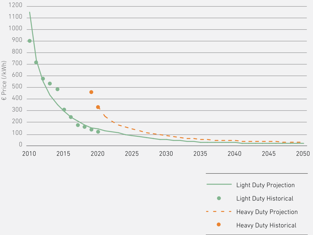
Batteriepreisszenarien für eLKW
