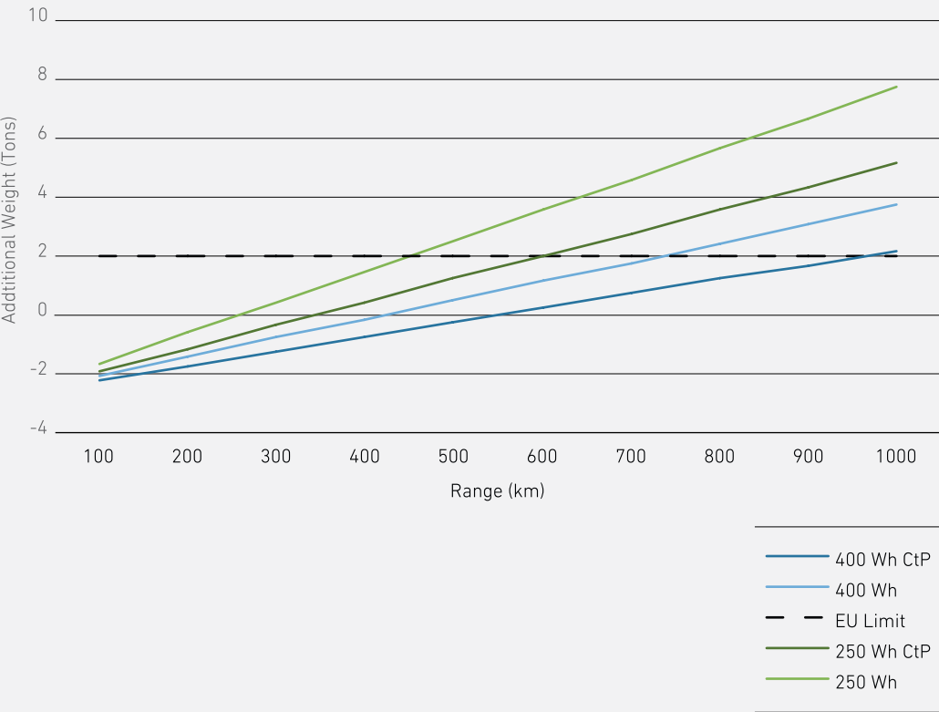
Mehrgewicht von eLKW mit zunehmender Reichweite und unterschiedlichen Energiedichten der Batteriezellen. Die Berechnung geht von einer Gewichtseinsparung von 2,7 t bei eLKW gegenüber Diesel-LKW aufgrund des leichteren Antriebsstrangs aus. Wh = Wattstunden; CtP = Cell-to-Pack
